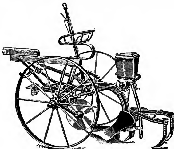
FIG. 3.—Maize Lister.
