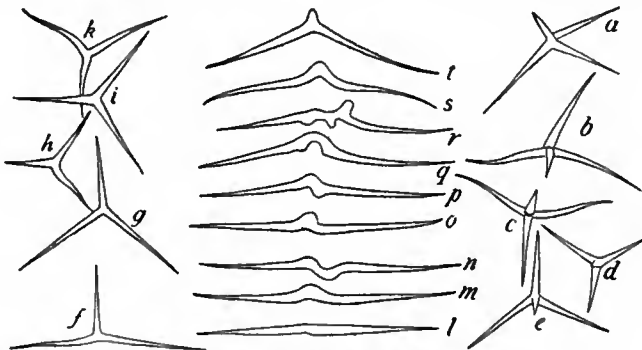
FIG. 5.— Plakina monolopha .
