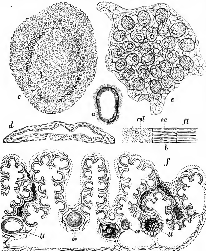
FIG. 4.— Plakina monolopha .
