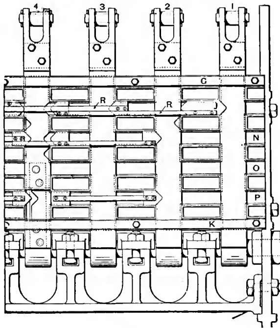
FIG. 7.—Interlocking Frame.
