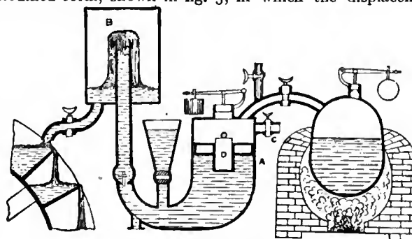
FIG. 3.—Papin, 1705.
