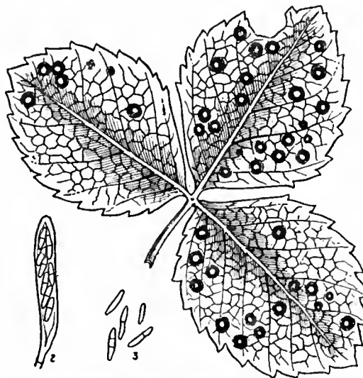
FIG. 3.— Sphaerella fragariae .
